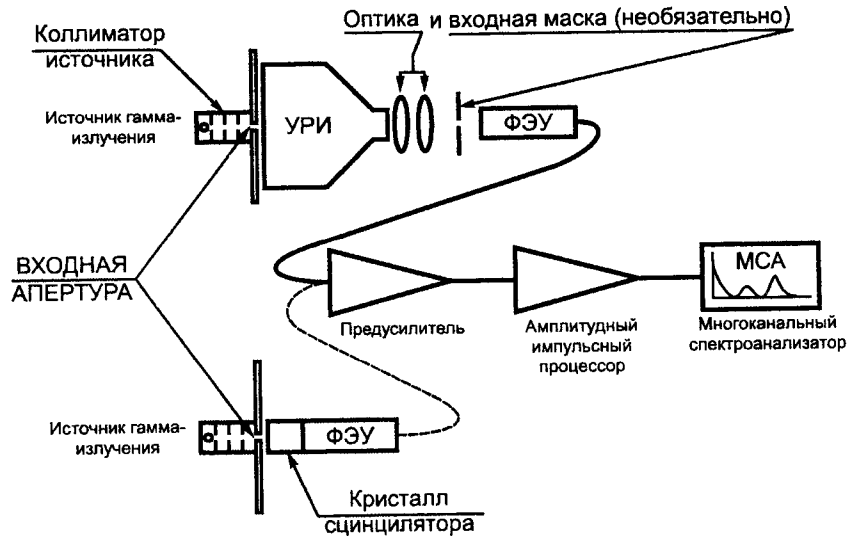
Типовая схема проведения испытаний
