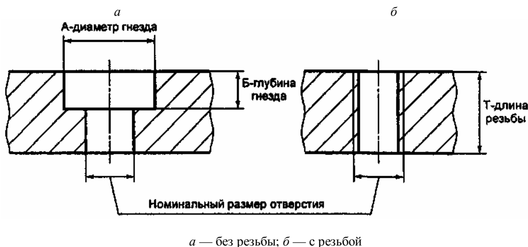
Рисунок 1 — Вспомогательные отверстия для крепления дополнительных деталей и устройств на корпусах и крышках задвижек
