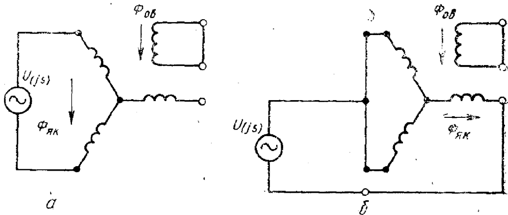
Продольная ось. Питание двух фаз обмотки якоря
