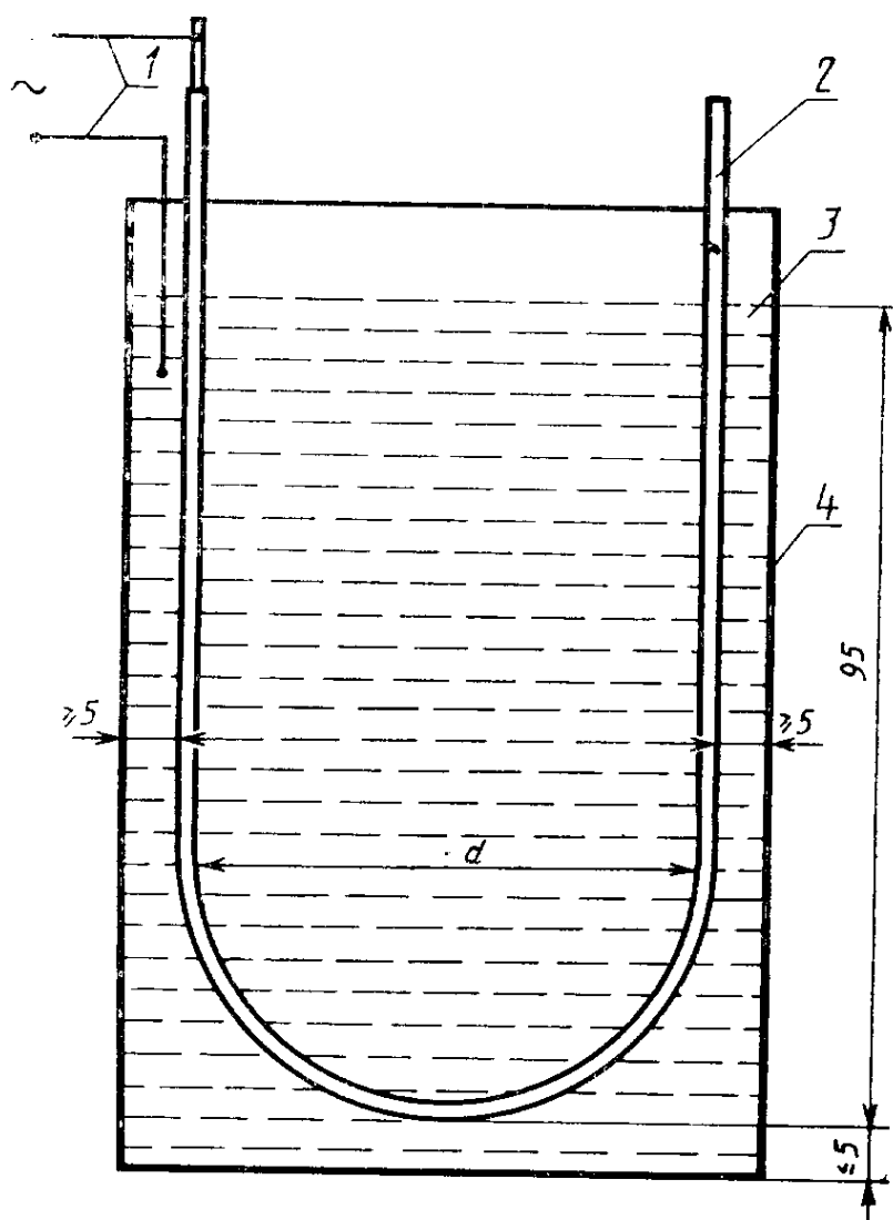
1—электроды; 2—испытуемый образец провода; 3—дробь; 4—ванна
