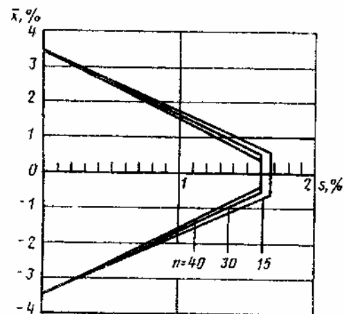
Метод \bar{x}, \bar{R}
