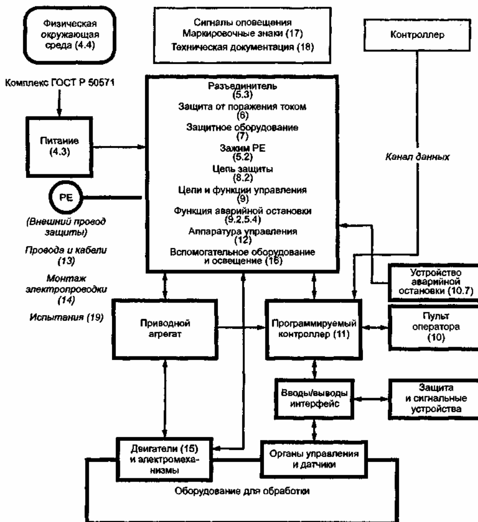
Рисунок 2 — Функциональная схема типовой машины
