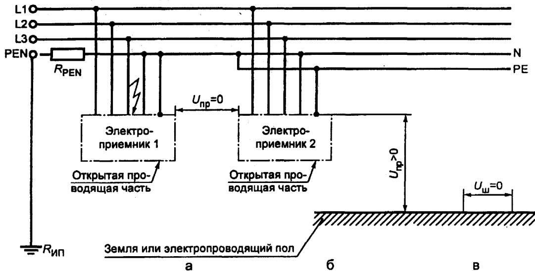
Рисунок В.9 — Сеть TN-C-S с однофазным замыканием на корпус до точки разделения PEN-проводника на N- и PE-проводники
