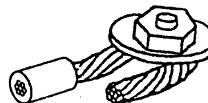
Рисунок F.2 — Косвенный зажим с помощью промежуточной детали неподготовленных проводников
