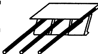
Рисунок F.6 — Примеры безвинтовых контактных зажимов
