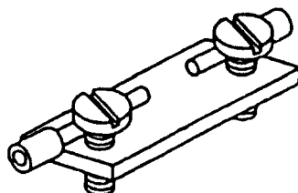
Рисунок F.1 — Непосредственный зажим головкой винта неподготовленных проводников
