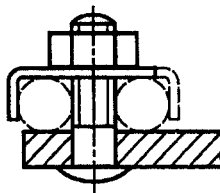
Рисунок F.2 — Косвенный зажим с помощью промежуточной детали неподготовленных проводников
