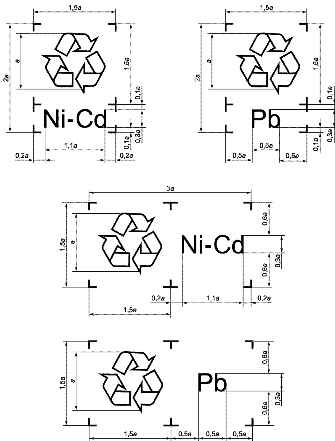
Рисунок 2 — Местоположение символов переработки и электрохимической системы батареи
