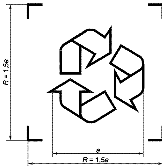
Рисунок 1 — Символ переработки ИСО 7000-1135 и площадь фоновой поверхности
