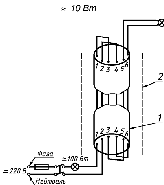
Рисунок 6 — Электрическая схема для испытания на нераспространение горения
