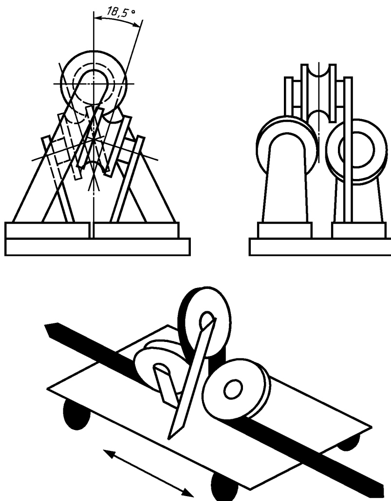
Рисунок 4 — Модифицированная каретка
