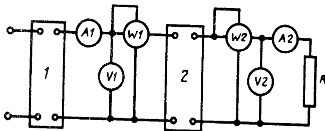
1 — регулятор напряжения; 2 — испытуемый трансформатор; R — номинальная нагрузка (резистор)
