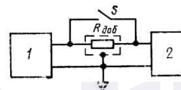
Схема определения входного сопротивления
