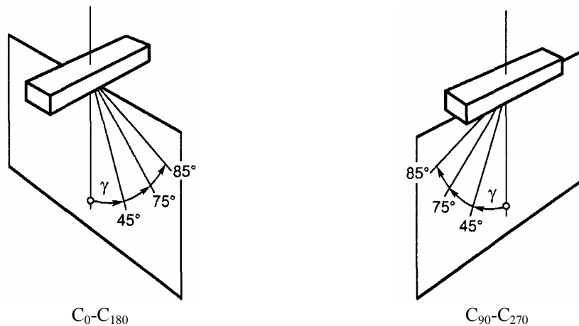
Рисунок А.4 — Плоскости С и углы \gamma , для которых должно быть проверено распределение яркости
